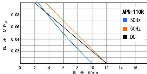
性能曲線 APN-110R
