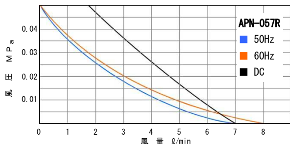
性能曲線 APN-057R
